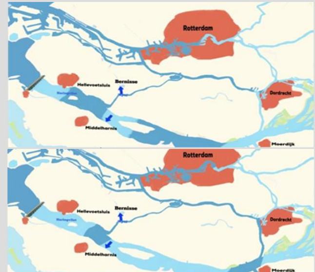
Figuur 4.4 Schematische weergave van het effect van een grotere ebopening op a) de waterstanden en daarmee b) de waterbeweging en zoutverspreiding in de Rijn-Maasmonding. NB. Omdat er geen berekeningen beschikbaar waren zijn de effecten op de waterstanden alleen schematisch weergegeven en niet verder gekwantificeerd
