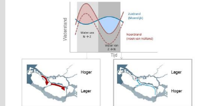
Figuur 2.3 Waterbeweging tussen noord en zuid onder extreme condities, zoals bijvoorbeeld peilopzet ten gevolge van wind
